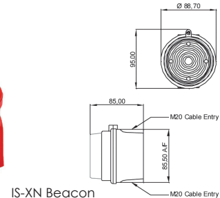
IS-XN Beacon
